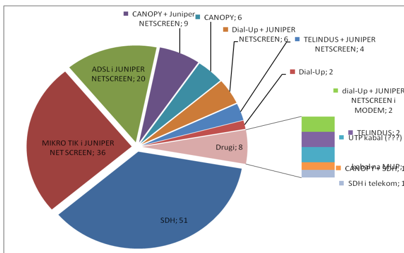
Grafikon broj 5 - Prikaz vrsta konekcija koju koriste izborna povjerenstva prilikom spajanja na aplikaciju „Pasivna registracija birača u BiH”
