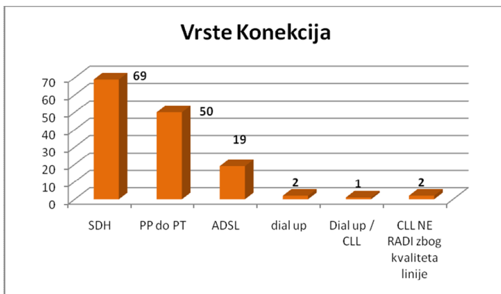
Графикон бр.7 - Врсте и број конекција које користе општинске изборне комисије
