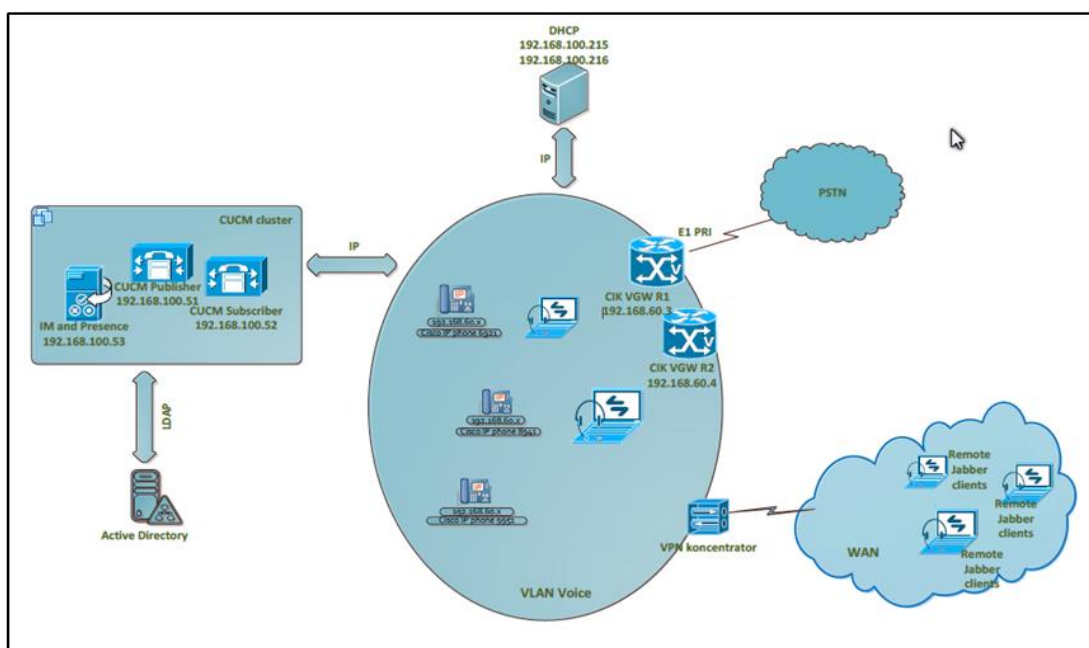
Slika 8. Prikaz IP telefonskog sustava
