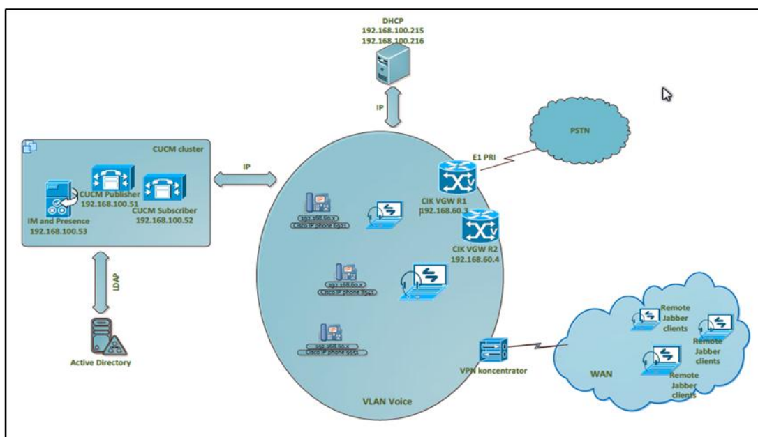
Слика 8. Приказ ИП телефонског система
